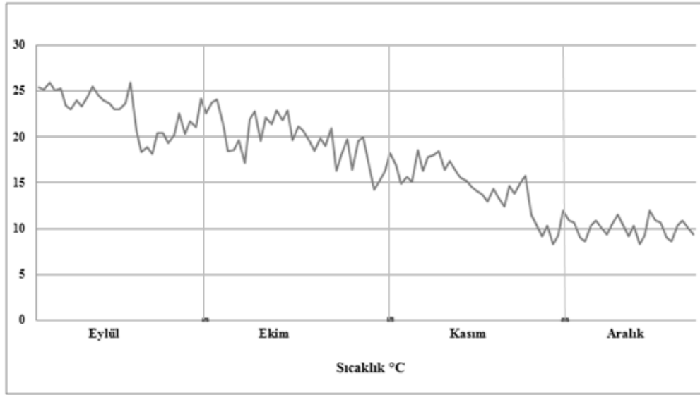
Şekil 1. Isıtmasız serada Eylül-Aralık yetiştirme dönemine ait ortalama sıcaklık değerlerinin günlük değişimleri
