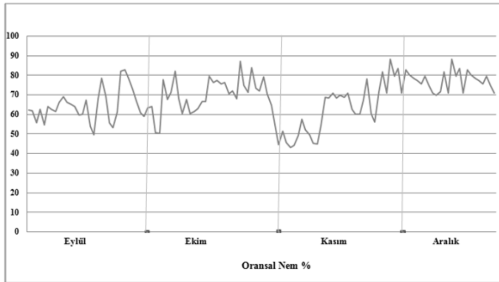
Şekil 2. Isıtmasız serada Eylül-Aralık yetiştirme dönemine ait ortalama oransal nem değerlerinin günlük değişimleri
