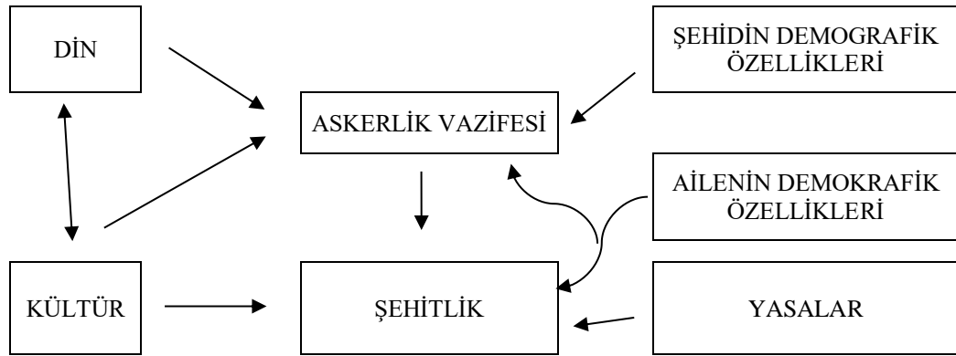
Şekil 1. 1. Araştırmanın Modeli
