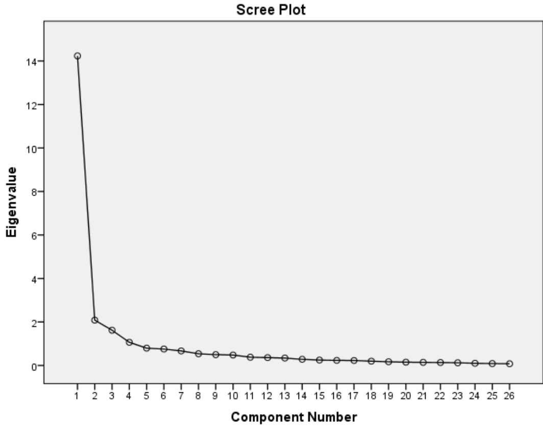
Şekil 4.1. Feminizme yönelik tutum ölçeğine ait yamaç grafiği
